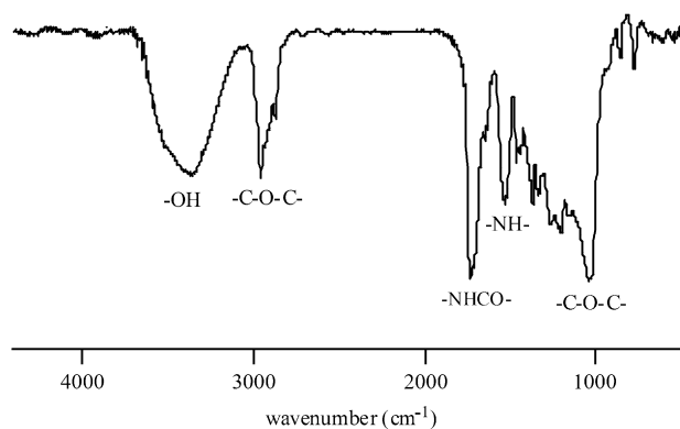
Fig. 2. IR spectrum of 3a (KBr film).
